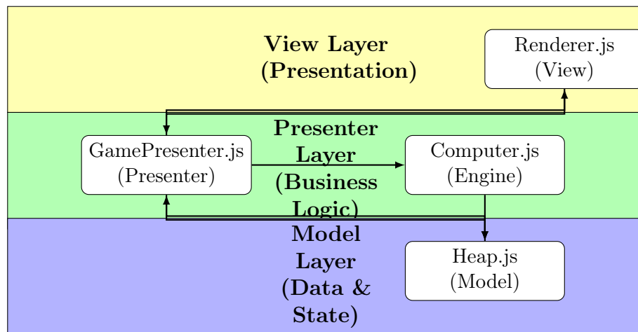
Figura 3.12: Diagramma Architetturale a Livelli (Layered Architecture)
