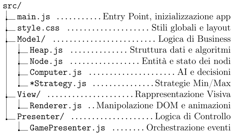
Figura 3.13: Struttura del File System del Progetto
